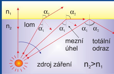
Obr. 3 a) úplný odraz, b) šíření světla v optickém vlákne
