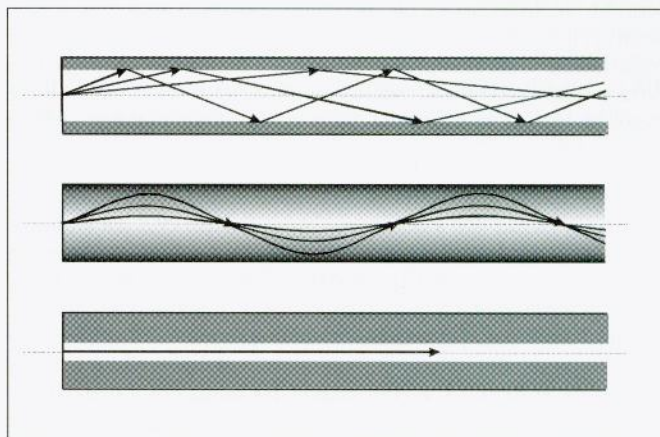
Obr. 3 Šíření paprsků v mnohovídrovém, gradientním a jednovídrovém vlákně. V důsledku různých optických drah různě skloněných paprsků nastává v mnohovídrovém vlákně rozšíření signálu (vidová disperze). V gradientním vlákně s vhodným radiálním gradientem indexu lomu k rozšíření nedochází, ale získání přesného gradientu je v praxi obtížné. Proto je nejvhodnější vlákno jednovídrové
